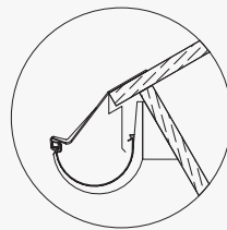
Fixatie voor T100
